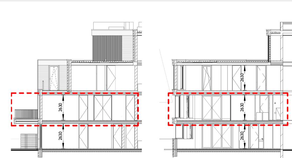
Doorsnede 1 - 1:200
