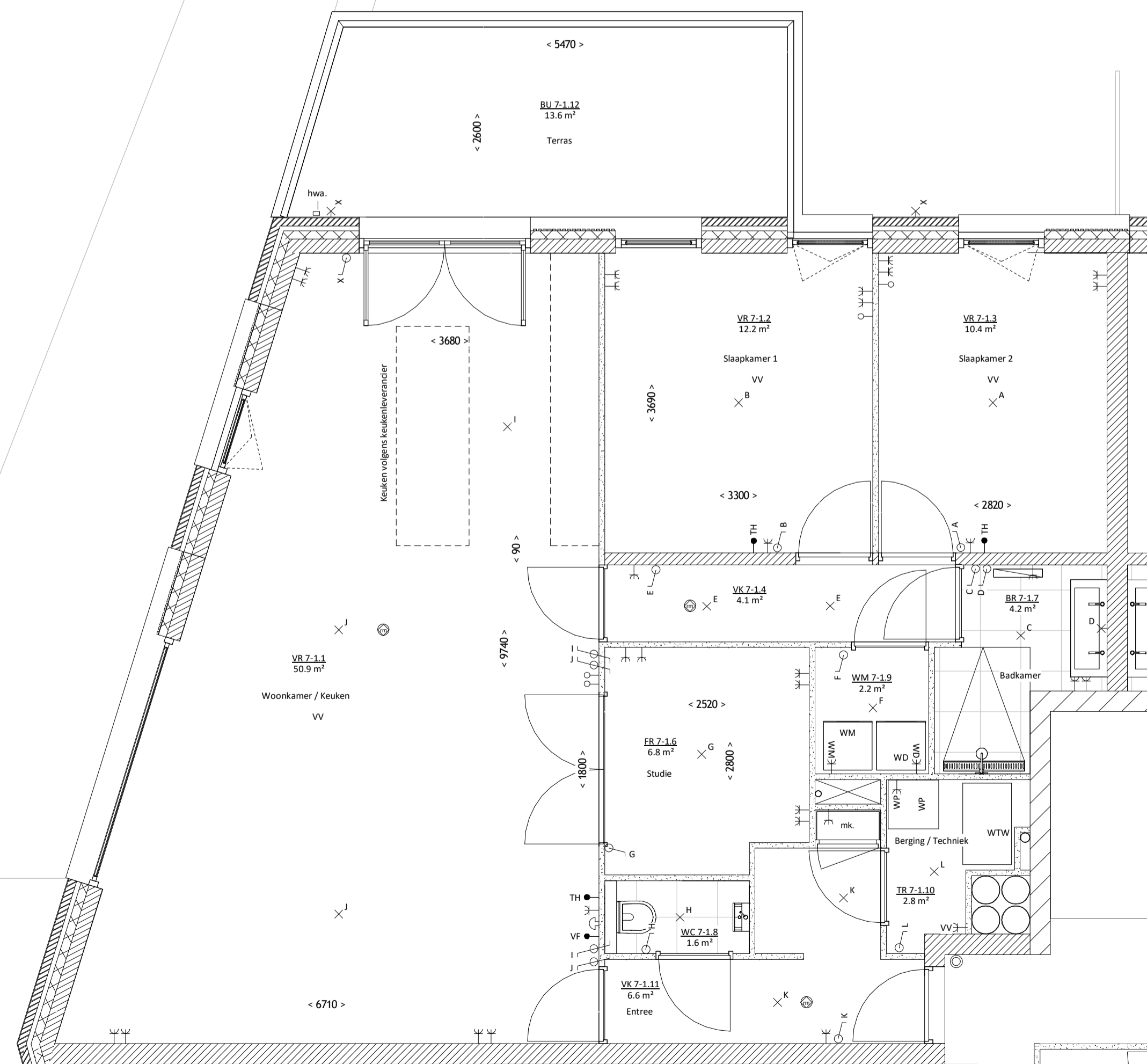
1e verdieping - 1:50
