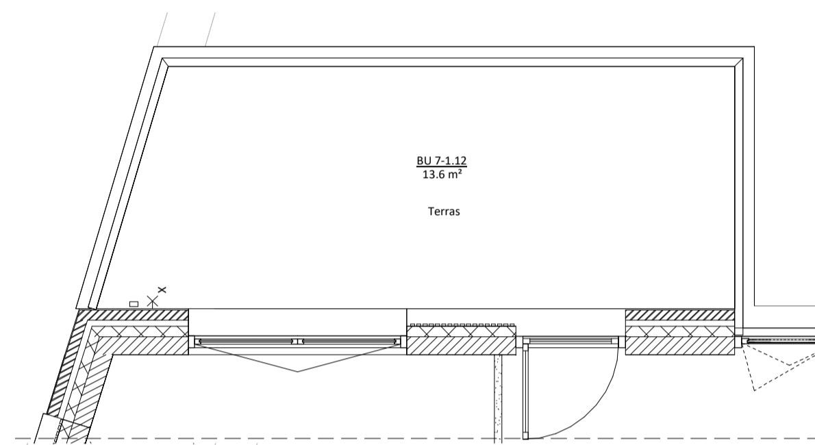
1e verdieping - 1:50 - optie
