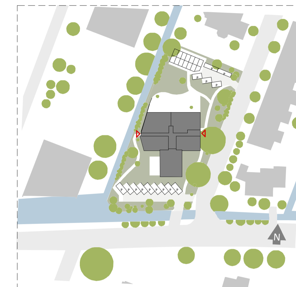
Situatie - 1:1000
