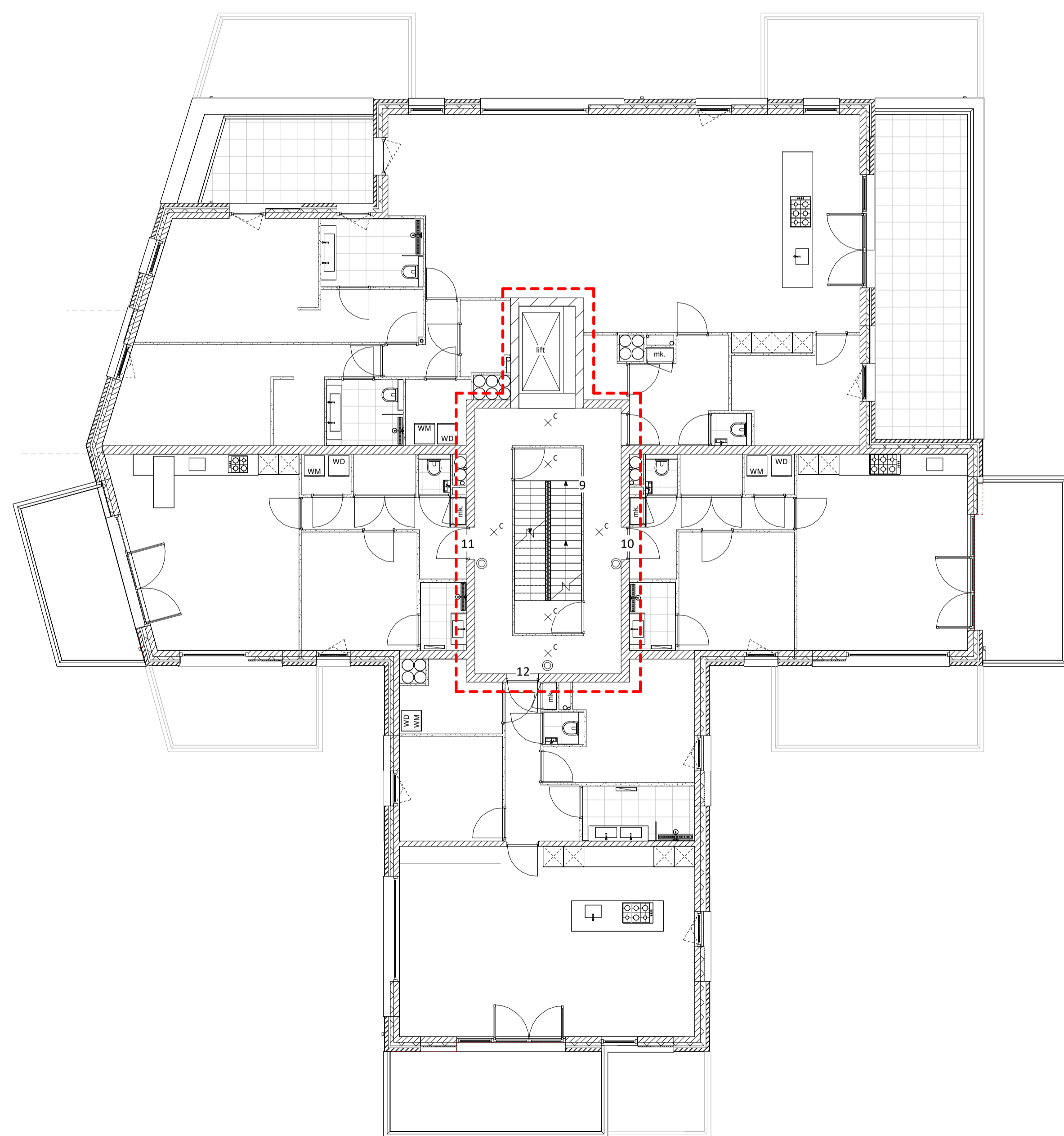
2e verdieping - 1:100
