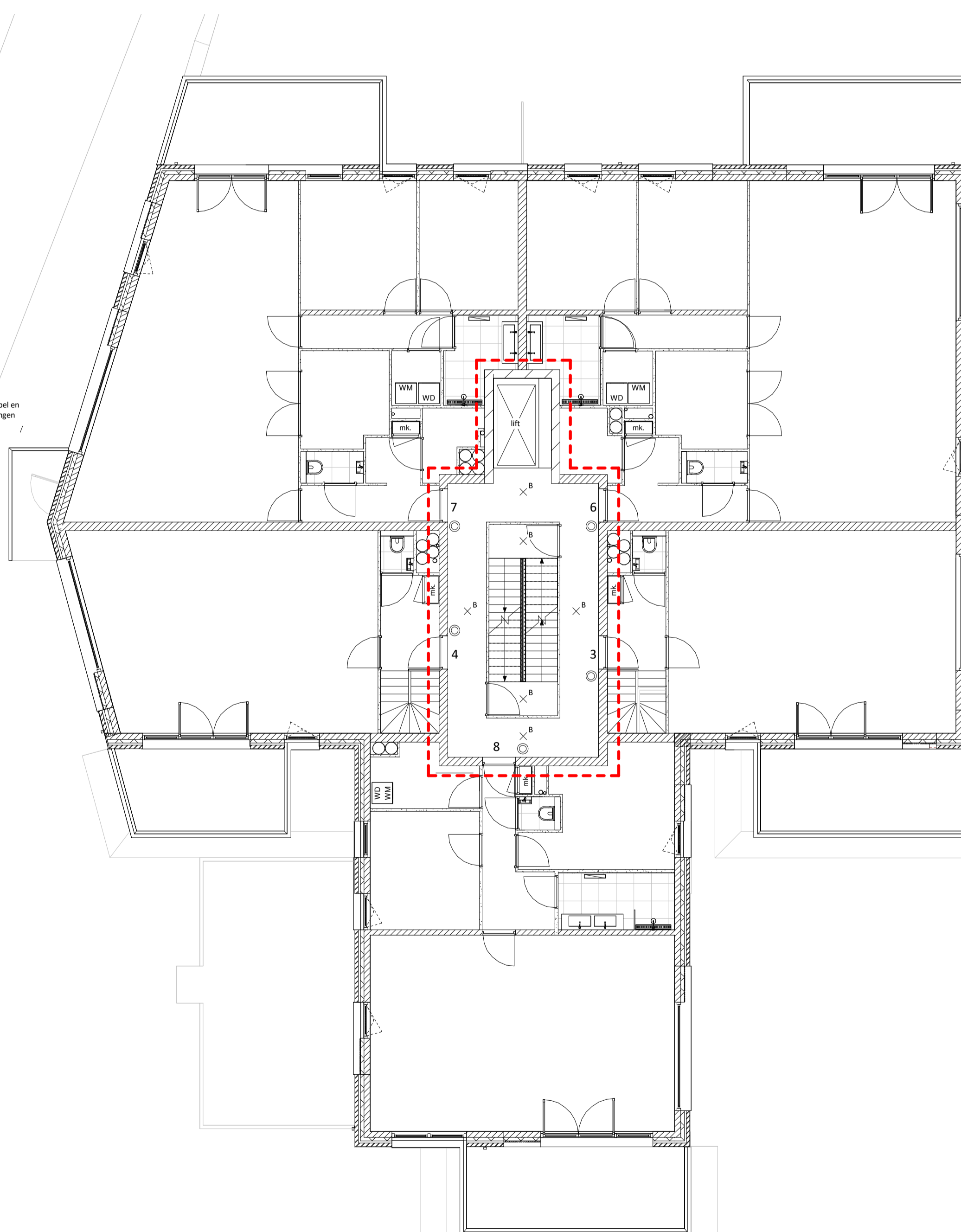
1e verdieping - 1:100
