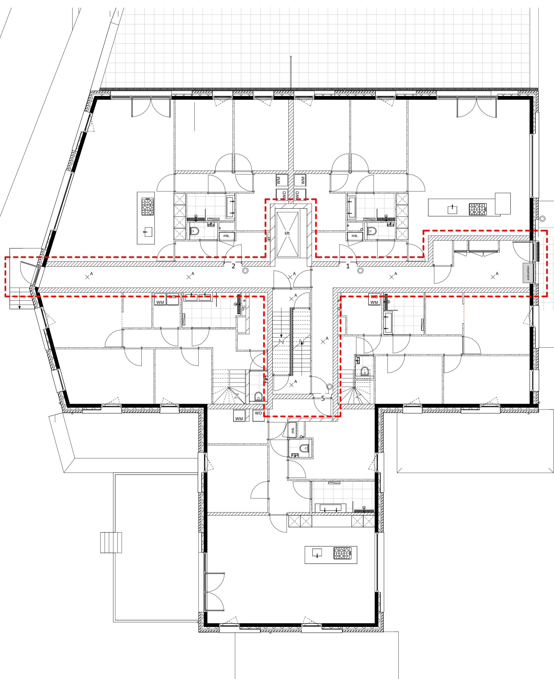
Begane grond - 1:100
